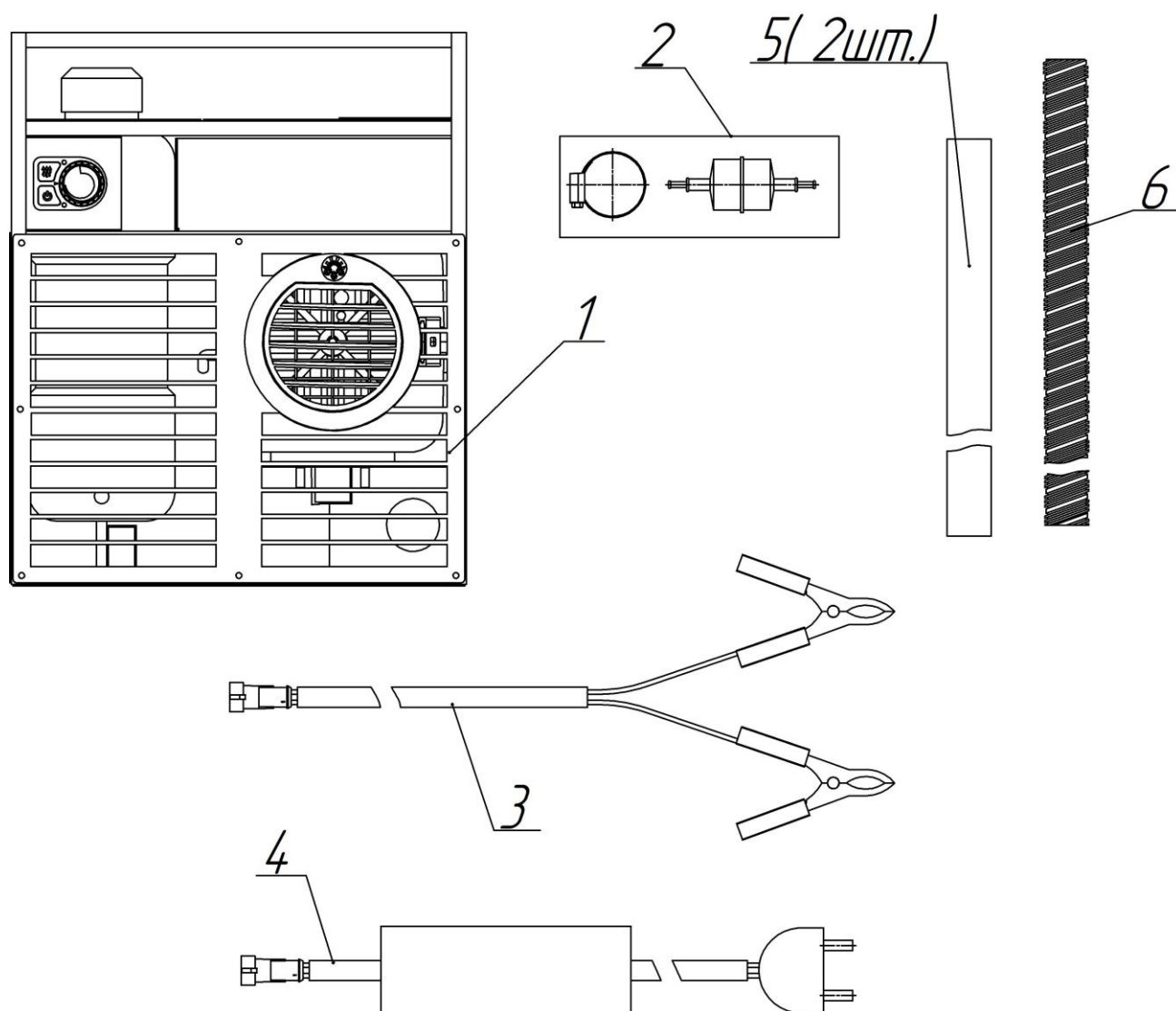
Рис.1- Комплект отопителя
